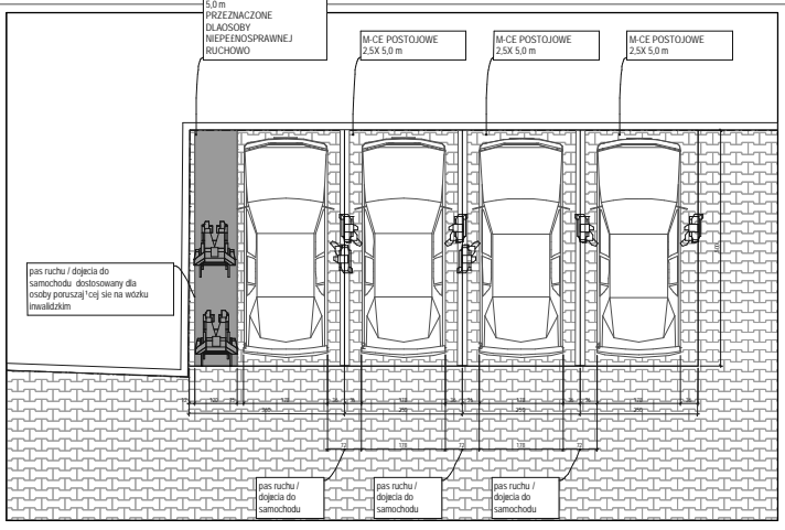
SZCZEGÓŁ ROZWIĄZAŃ MIEJSC POSTOJOWYCH PROJEKTOWANEGO PARKINGU
