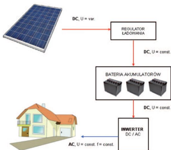
Rysunek 25. Schemat instalacji OFF-GRID 132 (oznaczenia: DC- prąd stały, AC-prąd przemienny, U- napięcie, f-częstotliwość, var.-zmienne, const.- stałe)
