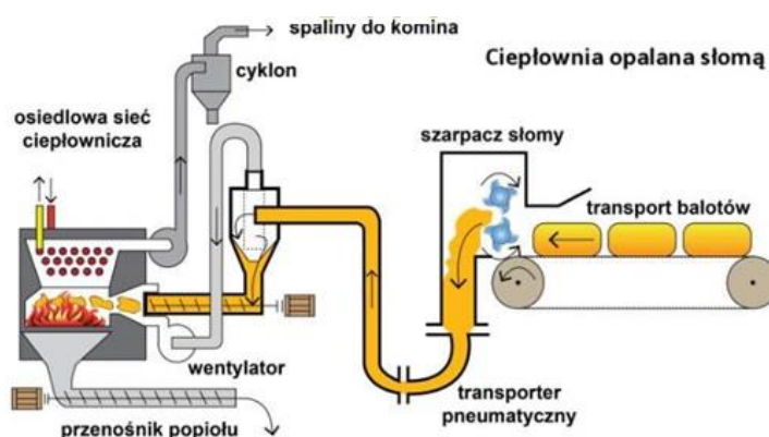
Rysunek 19. Schemat kotłowni na słomę 122
