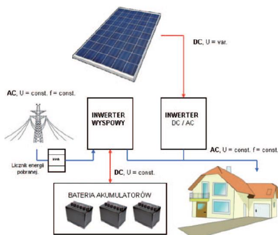
Rysunek 26. Schemat instalacji mieszanej 133 (oznaczenia: DC- prąd stały, AC-prąd przemienny, U- napięcie, f-częstotliwość, var.-zmienne, const.- stałe)
