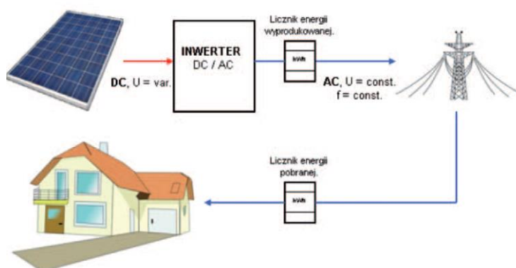
Rysunek 24. Schemat instalacji ON-GRID 131 (oznaczenia: DC- prąd stały, AC-prąd przemienny, U- napięcie, f-częstotliwość, var.-zmienne, const.- stałe)
